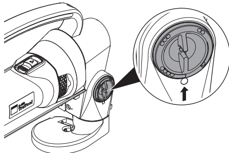
Εικ. 1: Ρυθμιστής ύψους μαχαιριού ωστηρίου
