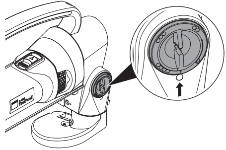
Рис. 1: Регулятор высоты подвижного ножа
