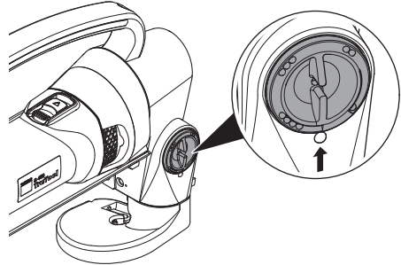
Abb. 1: Höhenregler Stößelmesser
