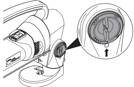
그림1: 조정식 커터 블레이드 높이 조절기
