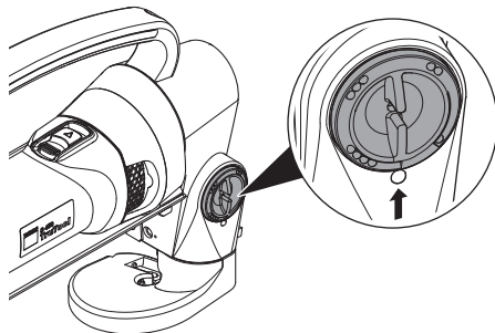
图1: 柱塞刀片高度调节器
